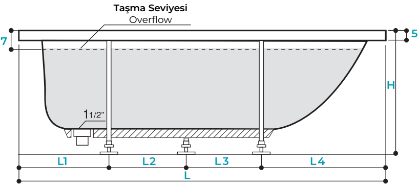
KESİT A-A SECTION A-A
