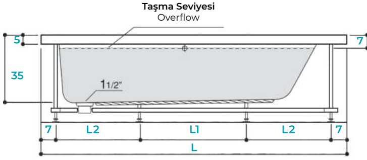
KESİT A-A SECTION A-A
