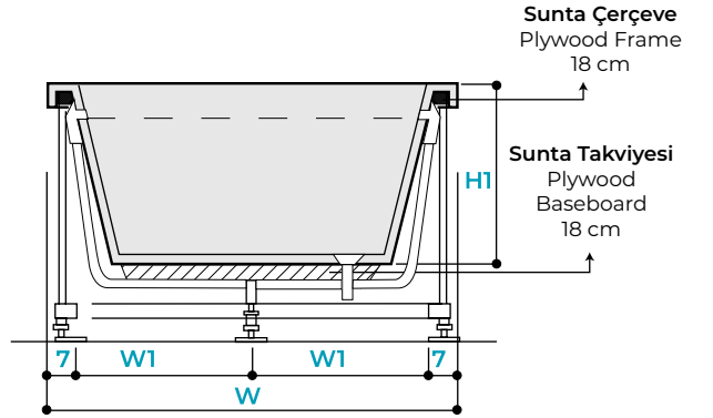
KESİT B-B SECTION B-B
