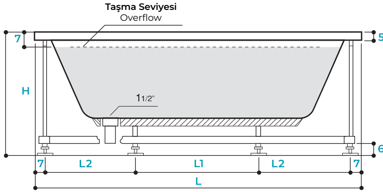
KESİT A-A SECTION A-A
