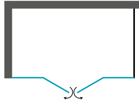
130 / 135 YP / SP 2 Sabit - 2 Açılır 2 Fixed - 2 Outward Opening
