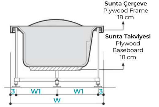
KESİT B-B SECTION B-B
