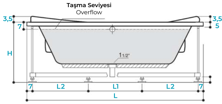
KESİT A-A SECTION A-A
