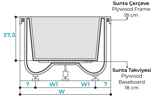
KESİT B-B SECTION B-B
