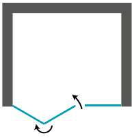
160 - D / O 1 Sabit 1 Katlanır 1 Fixed - 1 Outward Folding
