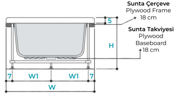
KESİT B-B SECTION B-B
