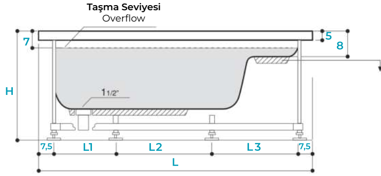
KESİT A-A SECTION A-A
