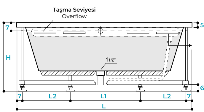
KESİT A-A SECTION A-A
