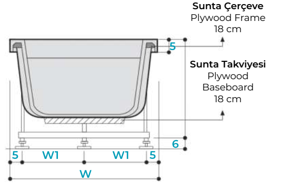
KESİT B-B SECTION B-B
