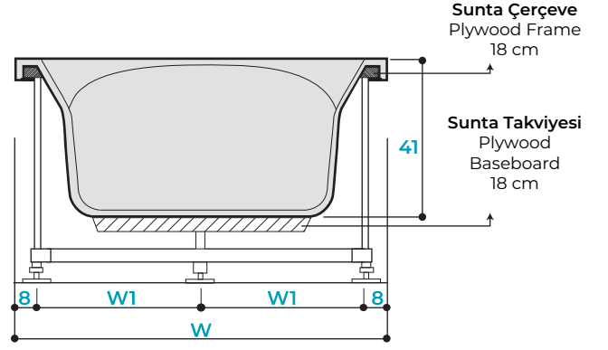
KESİT B-B SECTION B-B
